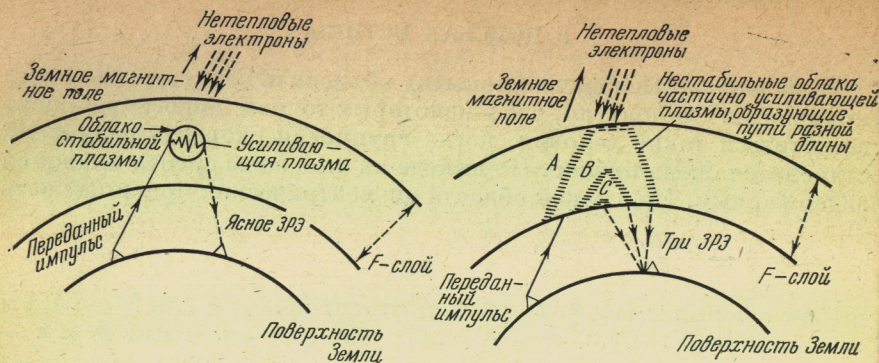
Рис. 10. Генерация «ясных» ЗРЭ в однородном стабильном плазменном облаке по [9]
