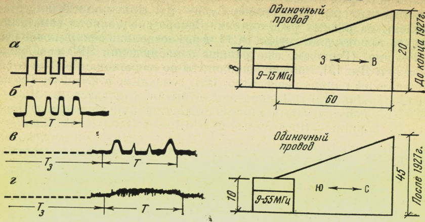
Рис. 3. Переданный и принятый радиосигналы станции РСJJ и два типа ЗРЭ а — передаваемый сигнал, символ «X», б — непосредственно принятый радиосигнал, задержка пренебрежимо мала; в — четкое эхо; г — размытое эхо. T = 2 с; T_3 = 1 \div 3 с — типичное время задержки
