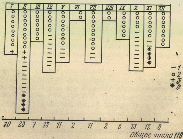
Рис. 12. Сезонный ход ЗРЭ по обобщенным данным с 1927 по 1973 г.
