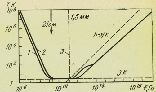
Рис. 2. Частотная зависимость яркостной температуры космического электромагнитного фонового излучения
