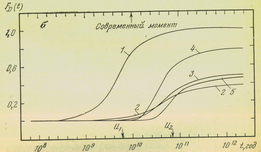
Рис. 4. Временной фактор (а) и полная вероятность возникновения коммуникативной цивилизации (б) для различных параметров (\theta_1, \theta_2) равномерного распределения времени развития T_0
