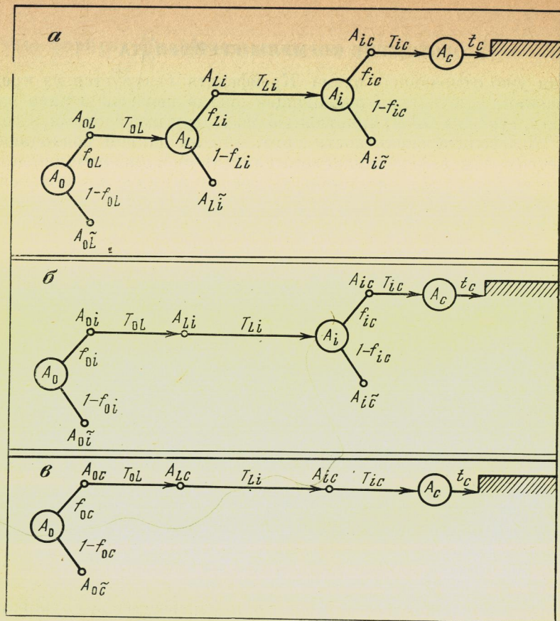
Рис. 2. Схема перехода подходящей звезды A_0 в коммуникативную фазу. Эта фаза отмечена штриховкой
