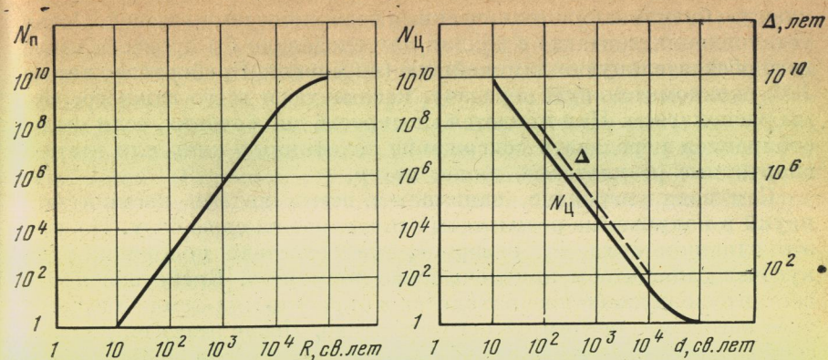
Рис. 1. Число звезд, «пригодных для обитания» N_{\Pi} в сфере радиуса R
