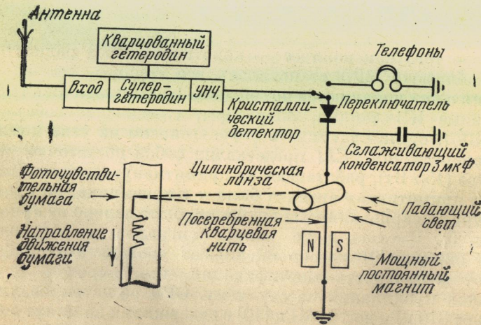
Рис. 5. Радиоприемное регистрирующее устройство Королевского колледжа в Лондоне
