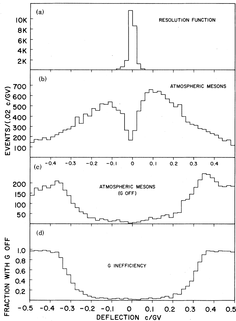
FIG. 1. Calibration data.
